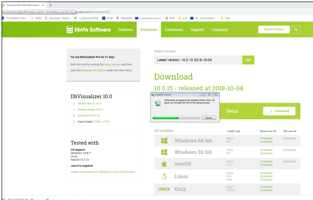
Fig. 8. DbVisualiser
